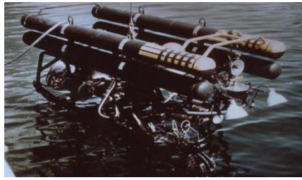
شکل شماره ۱: ربات XN-۳
