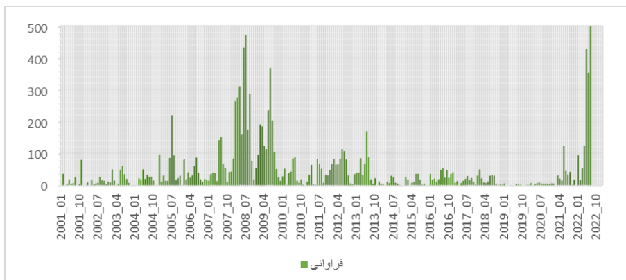
نمودار ۲: فراوانی طوفان‌های گردوخاک در بازه زمانی ۲۰۰۱-۲۰۲۳
