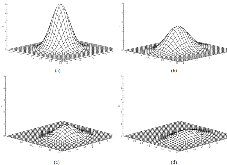
شکل ۲: میزان غلظت آلاینده در لحظات T=10 (a)، T=20 (b)، T=50 (c)، T=80 (d)
