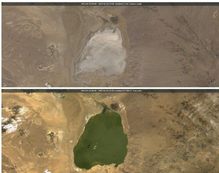
شکل ۱: مقایسه تالاب گاوخونی عکس ماهواره‌ای بالا ۱۴۰۱- پایین ۱۳۷۱ ( https://zayandehrud.com )
